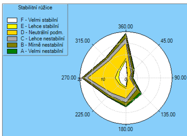
Obrázek 11 Stabilitní růžice
